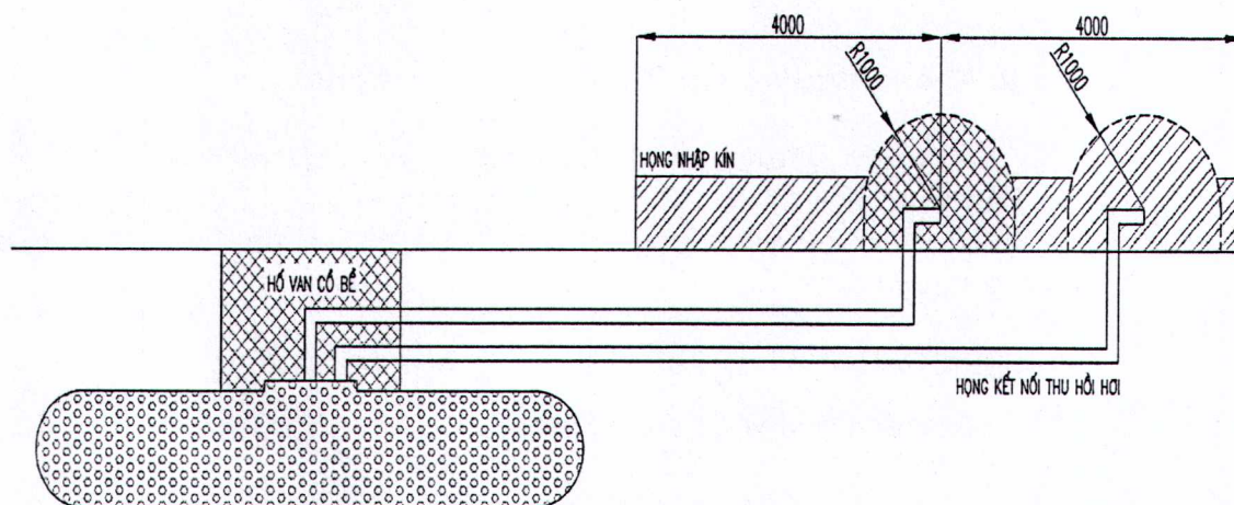
Hình 4: Vùng nguy hiểm cháy nổ bể chứa ngầm, hòng nhập kín và hòng thu hồi hơi xa vị trí cỏ bể và không đặt trong hố thao tác.
