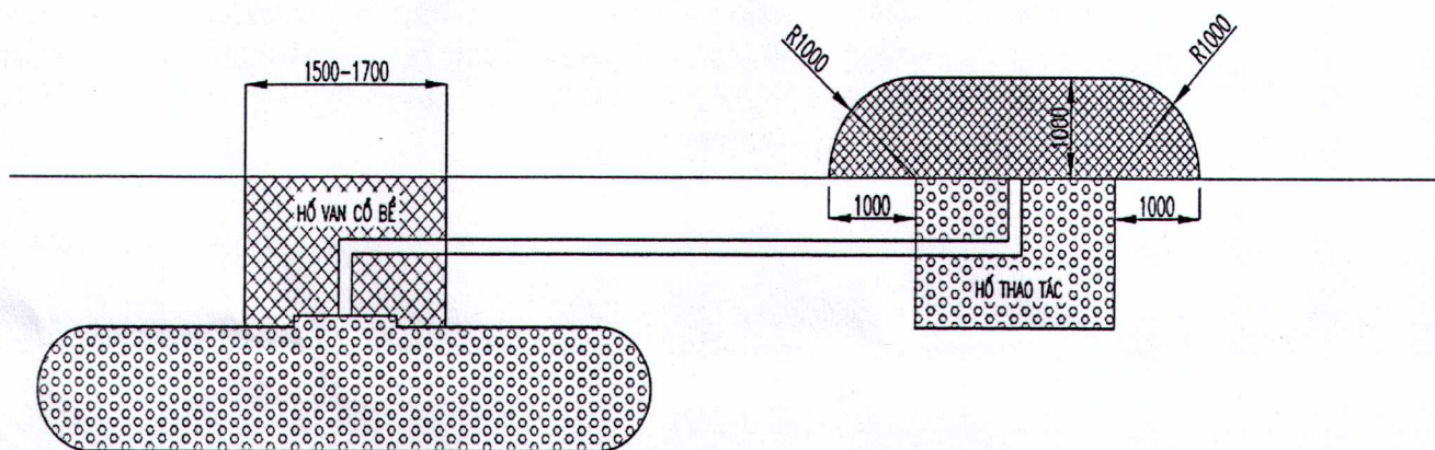
Hình 3: Vùng nguy hiểm cháy nổ bể chứa ngầm, hòng nhập kín và hòng thu hồi hơi xa vị trí cỏ bể và đặt trong hố thao tác.
