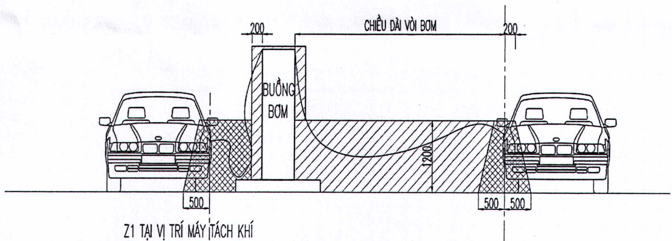
Hình 8: Vùng nguy hiểm cháy nổ xung quanh vị trí cột bơm khi đàn bán hàng cho phương tiện giao thông.
