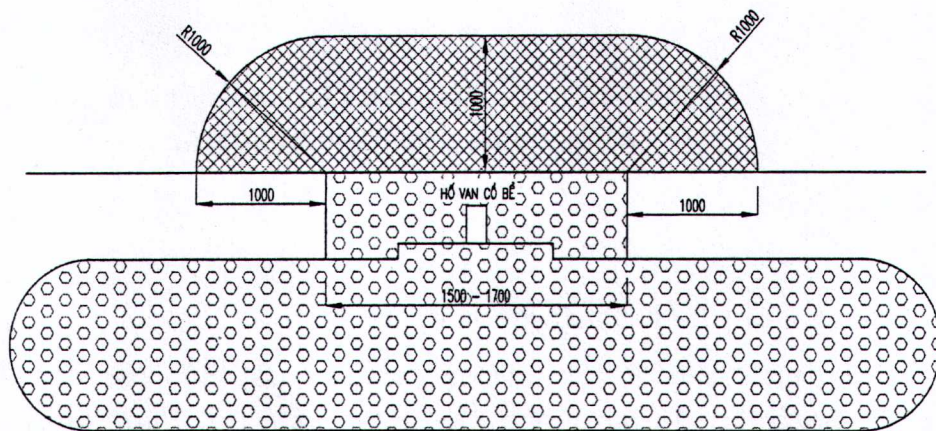
Hình 2: Vùng nguy hiểm cháy nổ bể chứa ngầm, hòng nhập kín và hòng thu hồi hơi ngay tại vị trí cỏ bể và đặt trong hố thao tác.
